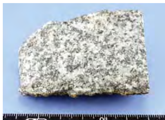
GR-37 輝石角閃石花崗閃緑岩 Pyroxene-Biotite Granodiorite
