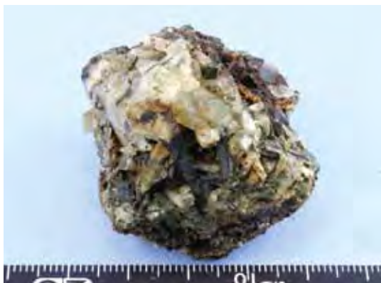
GR-17 石英 Quartz
