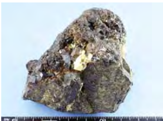
GR-20 ざくろ石 Garnet
