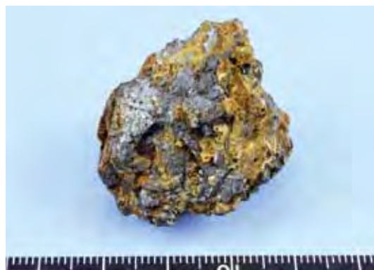
GR-14 磁鉄鉱 Magnetite
