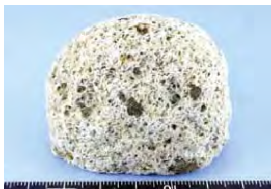
GR-66 流紋岩質軽石 Rhyolitic Pumice
